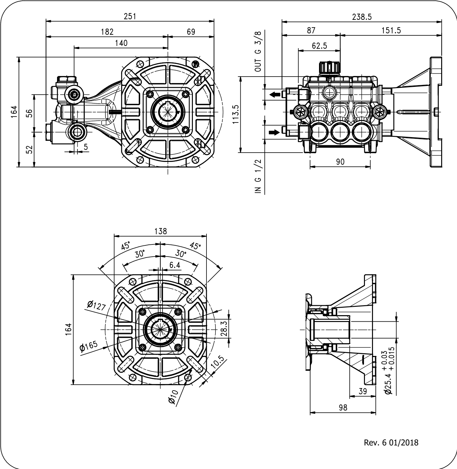
Dimensioni d'ingombro
