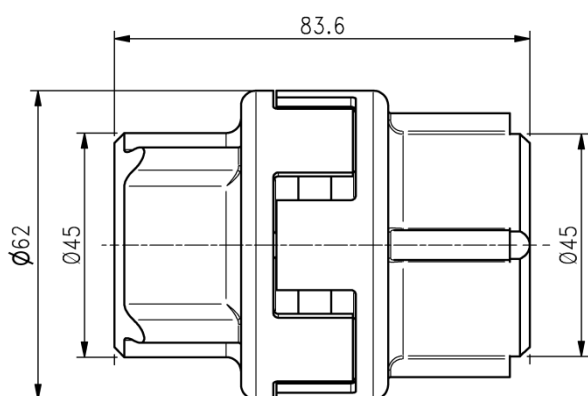
Attuali giunti flessibili serie NMT
