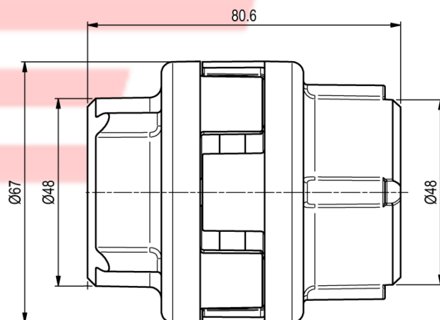
Nuovi giunti flessibili serie NHD
