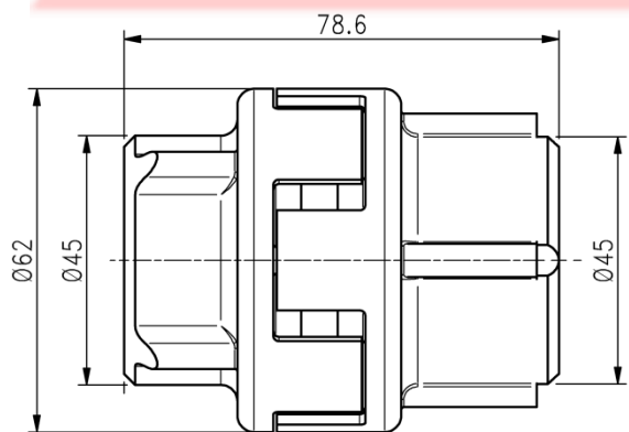
Attuali giunti flessibili serie NHD
